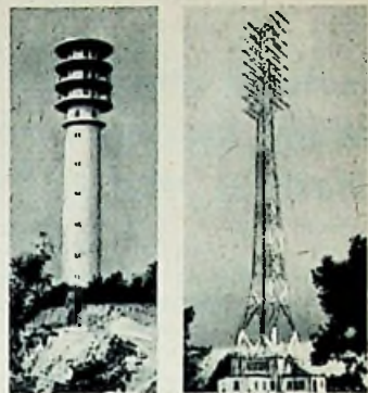
Twee relaisstations van het televisienet der NWDR. Links de 70 m hoge betontoren te Waldböhlen in de straalzenderverbinding Hamburg—Keulen en rechts de „klassieke” antennetoren van de tussenzender te Hühbeck aan de Elbe, in de koppeling Berlijn—Hamburg.
