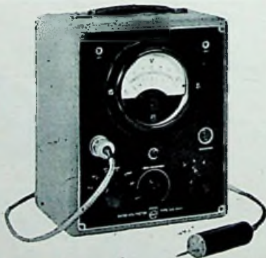
PHILIPS DIODE VOLTMETER Type GM 6004. Ideaal voor signal tracing.
